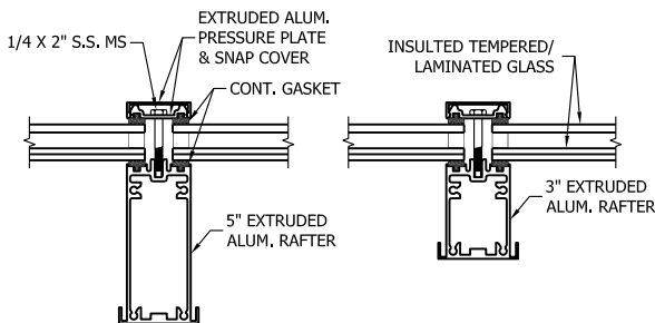
D RAFTER DETAIL SCALE: 3" = 1'-0"
