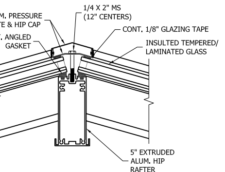
F HIP DETAIL SCALE: 3" = 1'-0"
